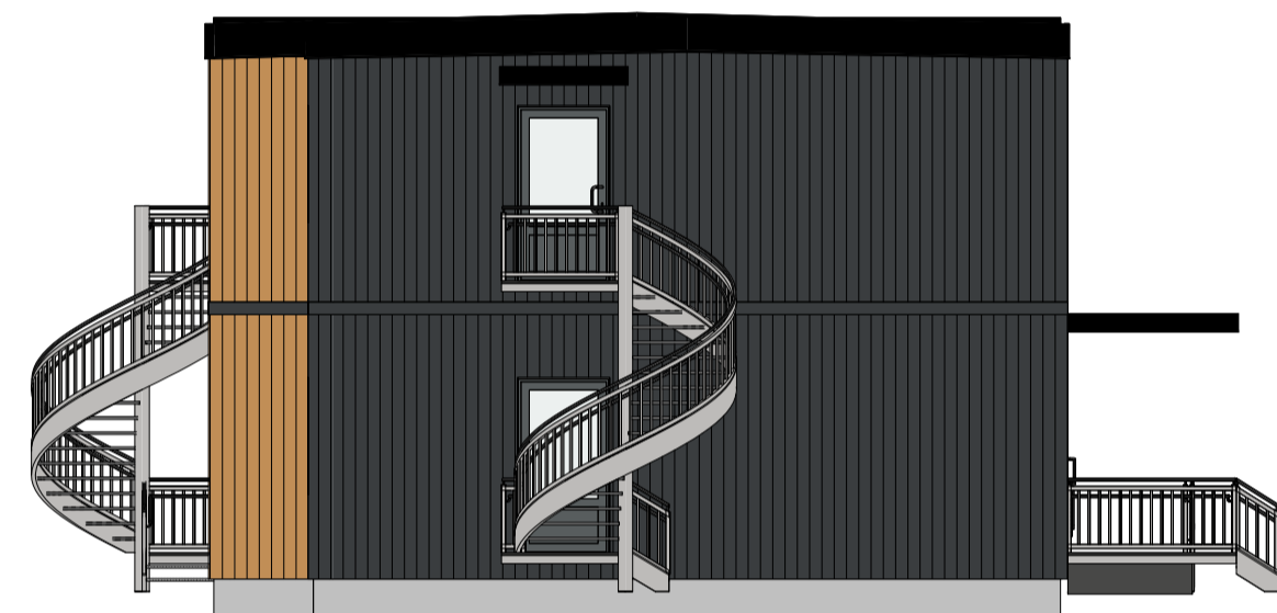
Vest 1 : 100
